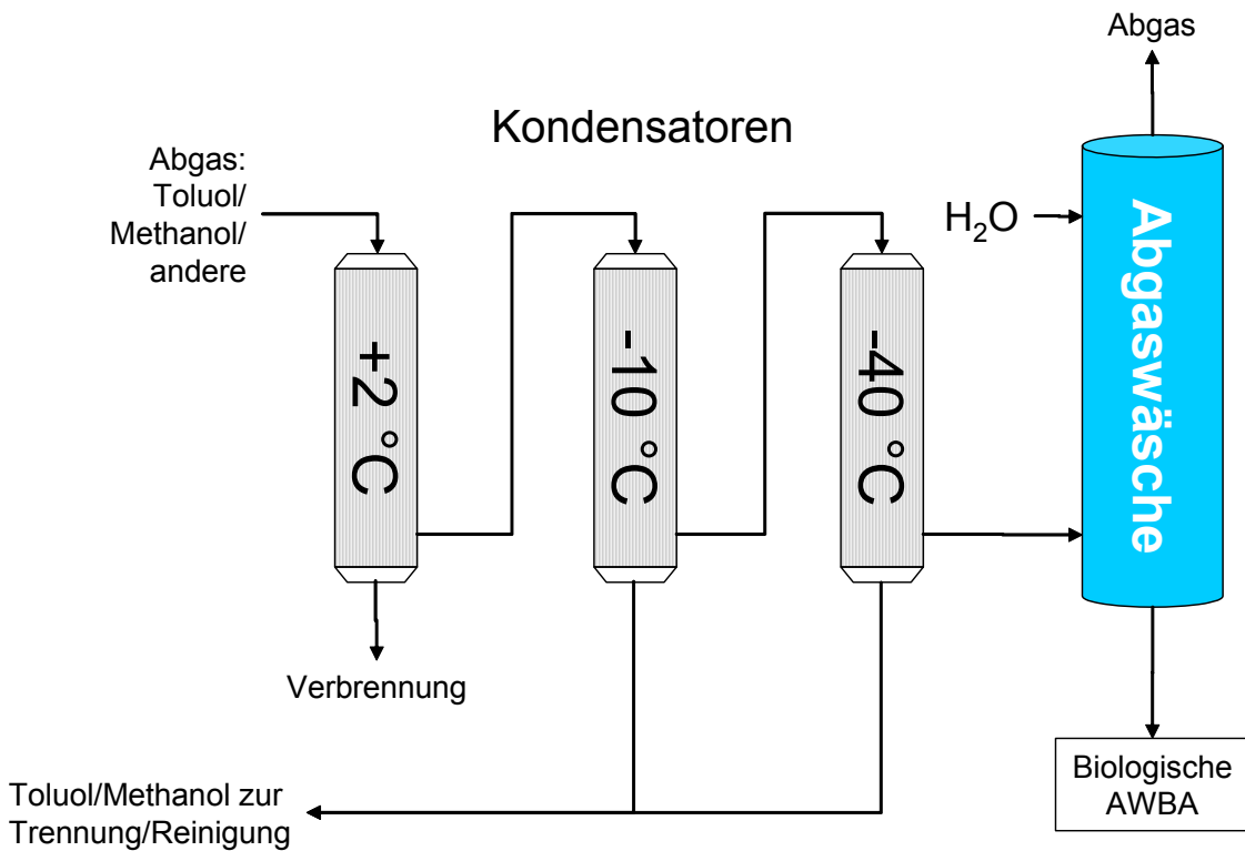
Abbildung 4.40: Rückgewinnung einer Toluol/Methanol-Mischung aus Abgasen
