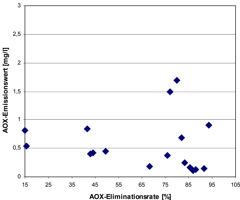
Abbildung 4.87: AOX-Eliminationsraten und -Emissionswerte
