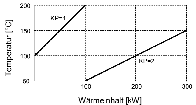
Abbildung 4.13: Zwei Wärmeströme
