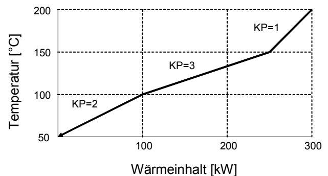
Abbildung 4.14: Warme Kompositkurve
