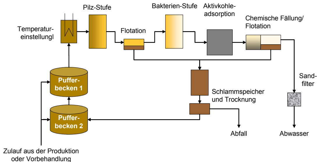
Abbildung 4.80: Behandlung des Gesamtabwassers mit zwei biologischen und einer Aktivkohlestufe
