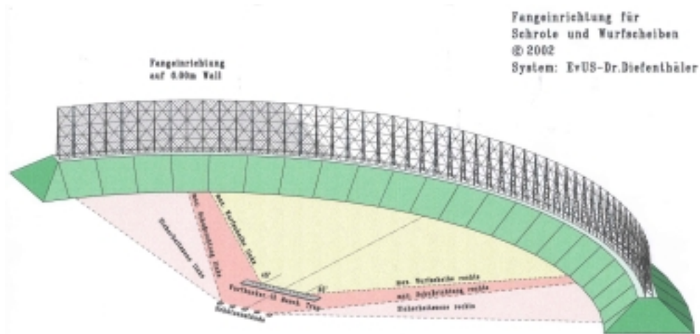
Abbildung 2: Wallanlage mit Schrottfanggitter
