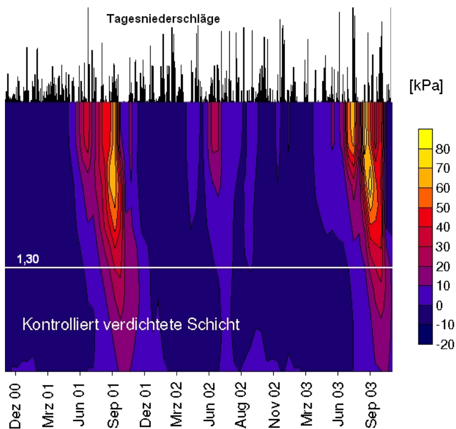
Abbildung 24 Wasserspannung in einer Rekultivierungsschicht Zeitlicher Verlauf in einem Beispiel Quelle: Ruhr-Universität Bochum, Prof. H. Zepp
