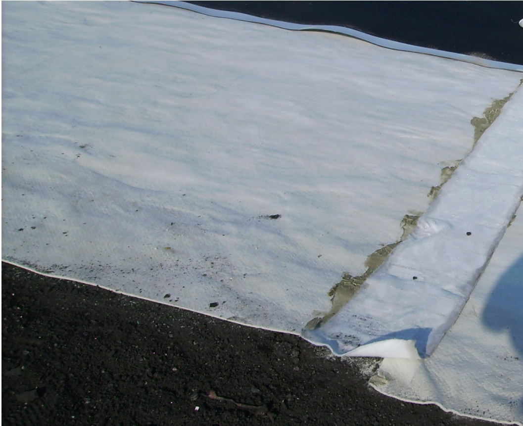
Abbildung 7 geosynthetische Tondichtungsbahn Überlappungszone (Querstoß) mit aufgetragener Bentonitpaste Foto: Naue GmbH & Co. KG
