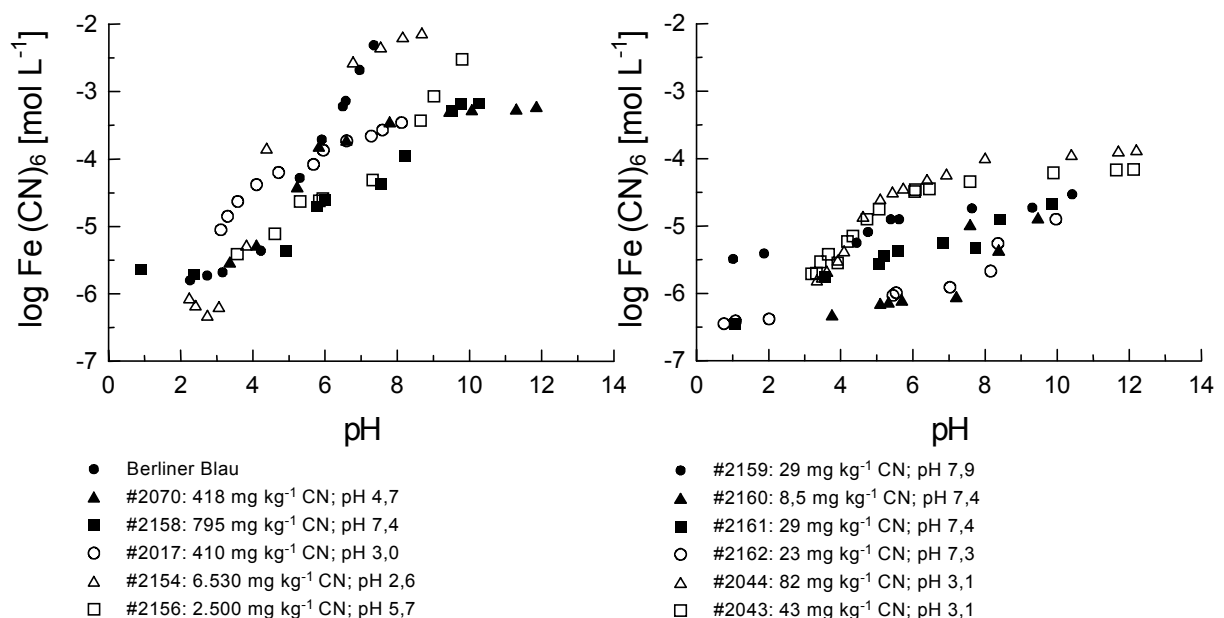
Abbildung 5.1 Beziehung zwischen dem pH -Wert und den Cyanid-Konzentrationen in 0,01 \text{ M CaCl}_2 -Extrakten von synthetischem Berliner Blau (links) und cyanidbelasteten Kokereiböden (links Böden mit > 100 \text{ mg CN kg}^{-1} ; rechts Böden mit < 100 \text{ mg CN kg}^{-1} ).
