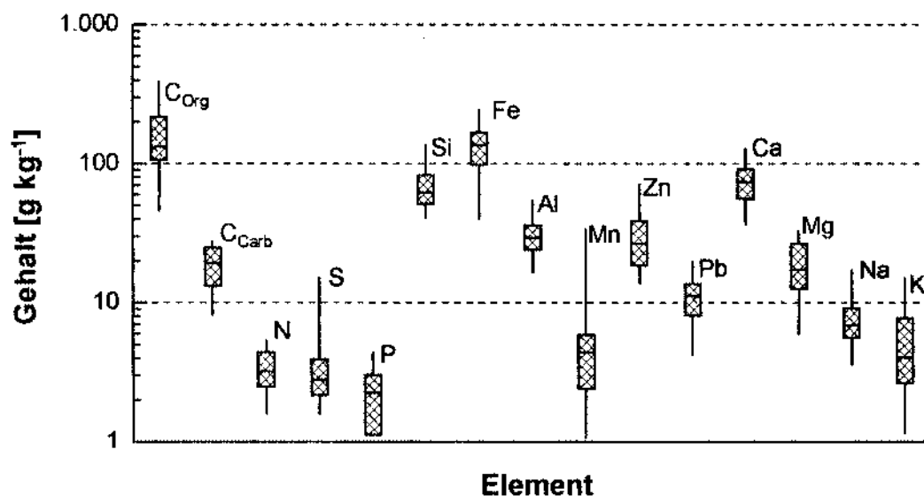
Abbildung 4.3 Elementarzusammensetzung von 32 Gichtgasschlammproben der Gichtgasschlamm-Deponie „Schalker Verein“ in Herne-Wanne, dargestellt mittels Box plots. Berücksichtigt sind nur Elemente mit Konzentrationen > 1 \text{ g kg}^{-1} .
