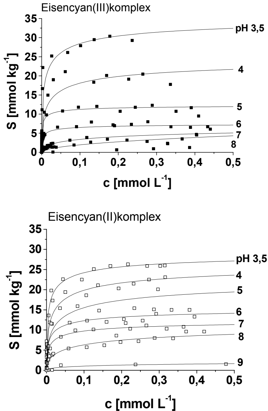
Abbildung 4.14 Sorption von Eisencyanokomplexen an Goethit in Abhängigkeit des pH -Wertes ( S = Sorptionsmaximum; c = Gleichgewichtskonzentration).
