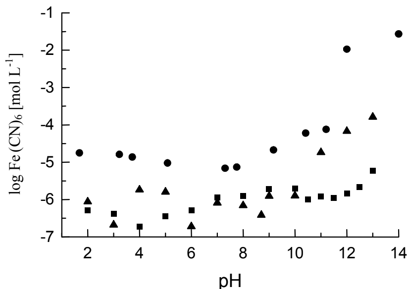
Abbildung 4.13 Einfluß vom \text{pH} -Wert auf die Cyanid-Konzentration in 0,01 \text{ M CaCl}_2 -Extrakten von Dikaliumtrizinkhexacyanoferrat(II) \cdot 9\text{H}_2\text{O} und von cyanidbelasteten Gichtgasschlämmen der Gicht-gasschlamm-Deponie „Schalker Verein“ in Herne-Wanne. (● \text{K}_2\text{Zn}_3[\text{Fe}(\text{CN})_6]_2 \cdot 9\text{H}_2\text{O} ; ■#2112; ▲#2125).
