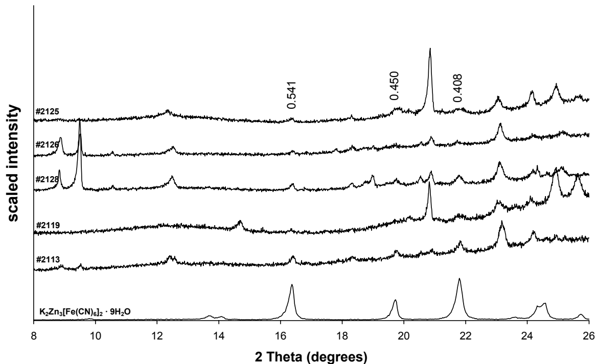
Abbildung 4.10 Pulver-Röntgendiffraktogramme von synthetisch hergestelltem K_2Zn_3[Fe(CN)_6]_2 \cdot 9H_2O und von fünf Gichtgasschlämmen mit unterschiedlichen Cyanidkonzentrationen der Gichtgasschlamm-Deponie „Schalker Verein“ in Herne-Wanne. #2113 = 7.400 mg CN kg -1 ; #2128 = 4.300 mg CN kg -1 ; #2126 = 2.750 mg CN kg -1 ; #2125 = 2.800 mg CN kg -1 . Einige der stärksten Reflexe mit den dazugehörigen d-Werten in nm sind aufgeführt.
