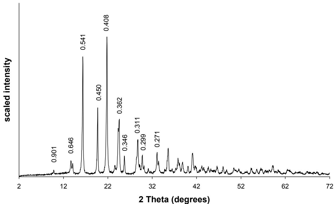
Abbildung 4.8 Pulver-Röntgendiffraktogramm von synthetisch hergestelltem K_2Zn_3[Fe(CN)_6]_2 \cdot 9 H_2O . Einige der stärksten Reflexe mit den dazugehörigen d-Werten in nm sind aufgeführt.
