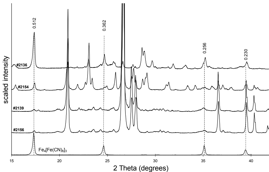
Abbildung 5.4 Pulver-Röntgendiffraktogramme von synthetisch hergestelltem Berliner Blau, \text{Fe}_4[\text{Fe}(\text{CN})_6]_3 , und von vier cyanidbelasteten Kokereiböden. #2136 = 63.200 \text{ mg CN kg}^{-1} ; #2154 = 6.530 \text{ mg CN kg}^{-1} ; #2139 = 2.510 \text{ mg CN kg}^{-1} ; #2156 = 2.500 \text{ mg CN kg}^{-1} . Das Berliner Blau-Diffraktogramm ist 0,2fach dargestellt. Einige der stärksten Reflexe mit den d-Werten in nm sind dargestellt.
